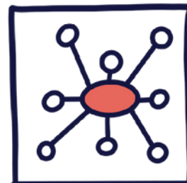
Mindmap
